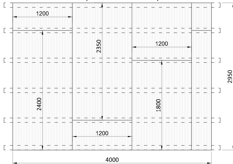
- Figura 6 – Capa inferior -tableros fibroyeso- (dimensiones en mm)
