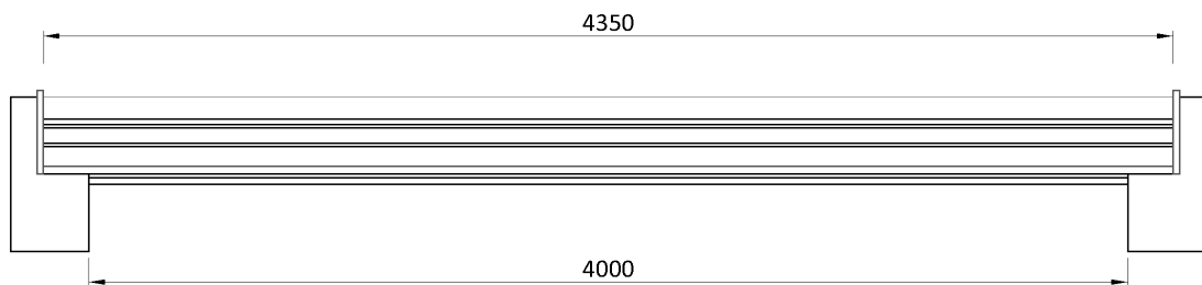
- Figura 2 – Esquema general de ensayo -sección longitudinal- (dimensiones en mm)
