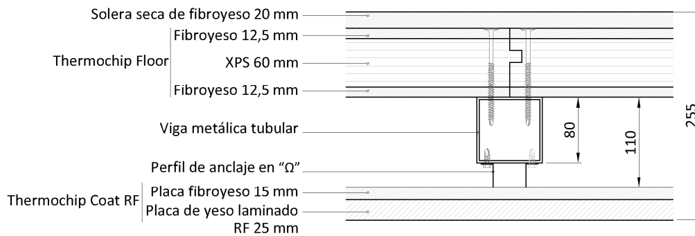
- Figura 3 – Sección transversal -detalle- (dimensiones en mm)
