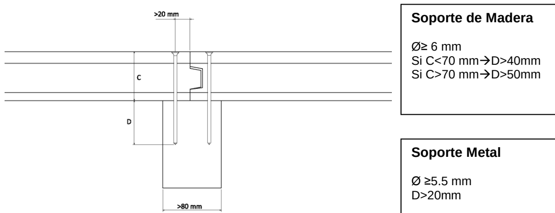
Figura 4. Fijaciones
