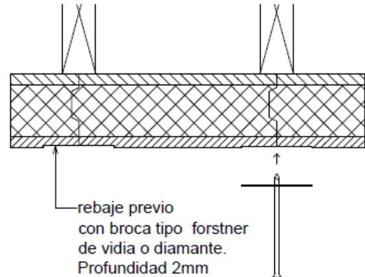
Instalación de tornillo con arandela (4,8 mm de diámetro y arandela de 40 mm de diámetro) con rebaje (hilera de borde vertical).
