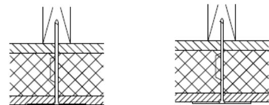
Tornillo con arandela (4,8 mm de diámetro y arandela de 40 mm de diámetro) con rebaje.
