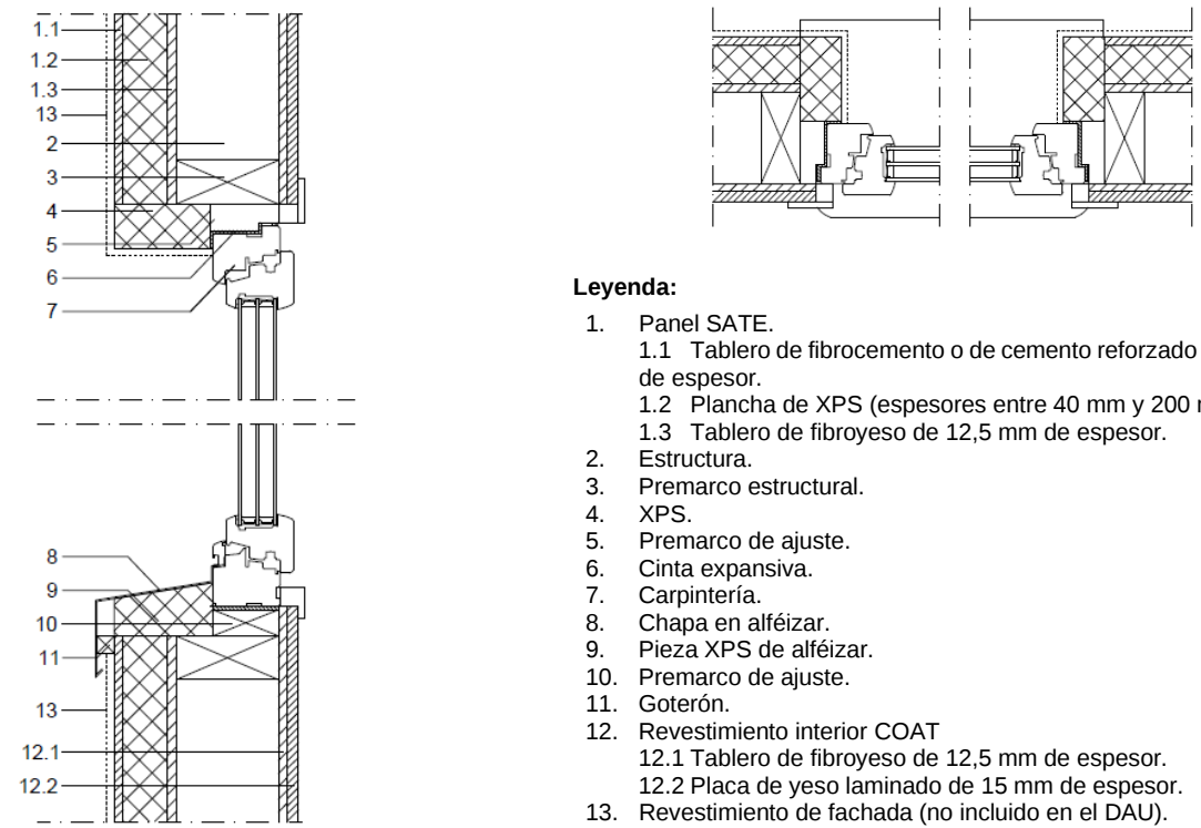
Figura 5.2: Encuentro tipo de fachada formada con paneles SATE y Revestimiento interior COAT con carpintería. Sección transversal horizontal y vertical.
