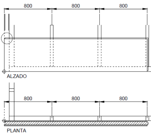
Figura 6.2: Colocación del primer panel y corte del machihembrado.
